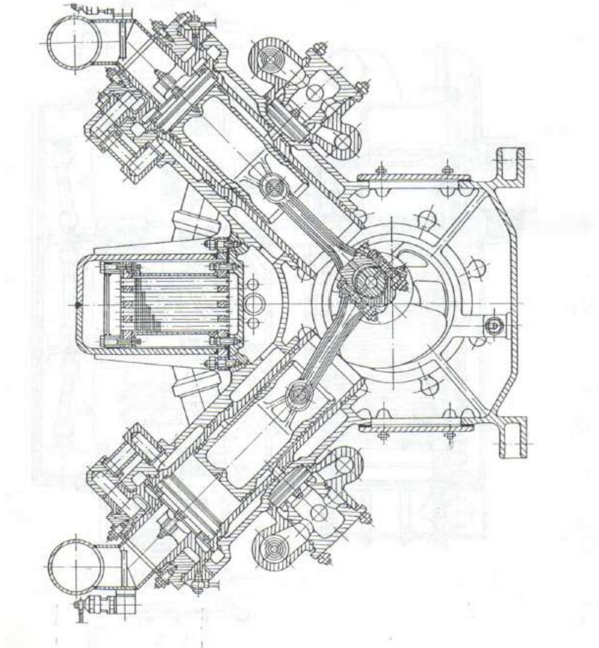
Przekrój poprzeczny sprężarki SFV6-125.
