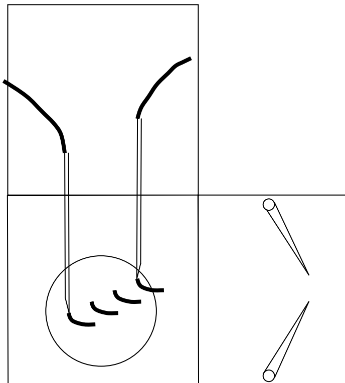
Rys. 2. Schemat układu tunelu w konfiguracjach roboczych: a – konfiguracja dla palisady sprężarkowej, b – konfiguracja dla palisady turbinowej.
