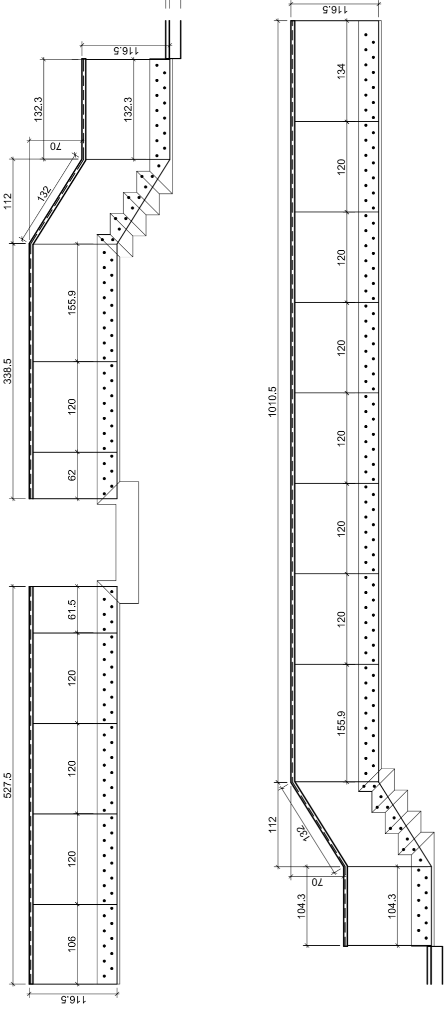
BALUSTRADA B1
